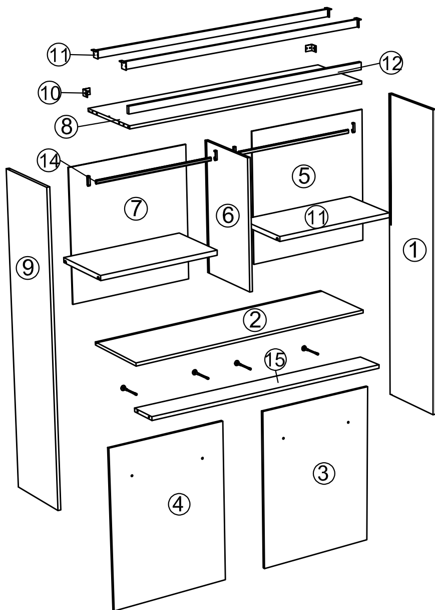
Ponte con schiena Brückenmodul mit Rückwand
