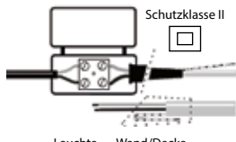
← Leuchte Wand/Decke →
