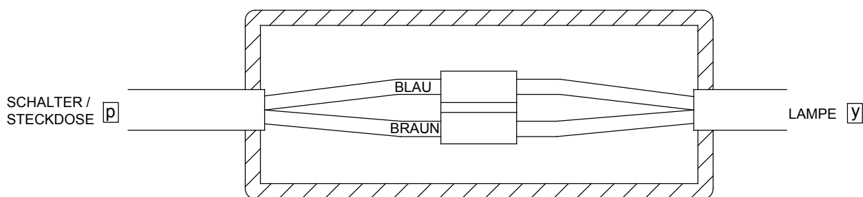
T16/ ANSCHLUSSDOSE
