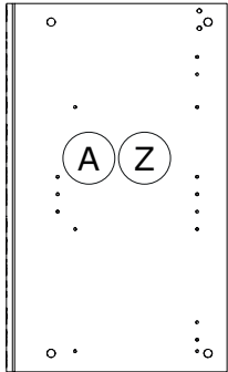
FI10141 676x405x16mm
