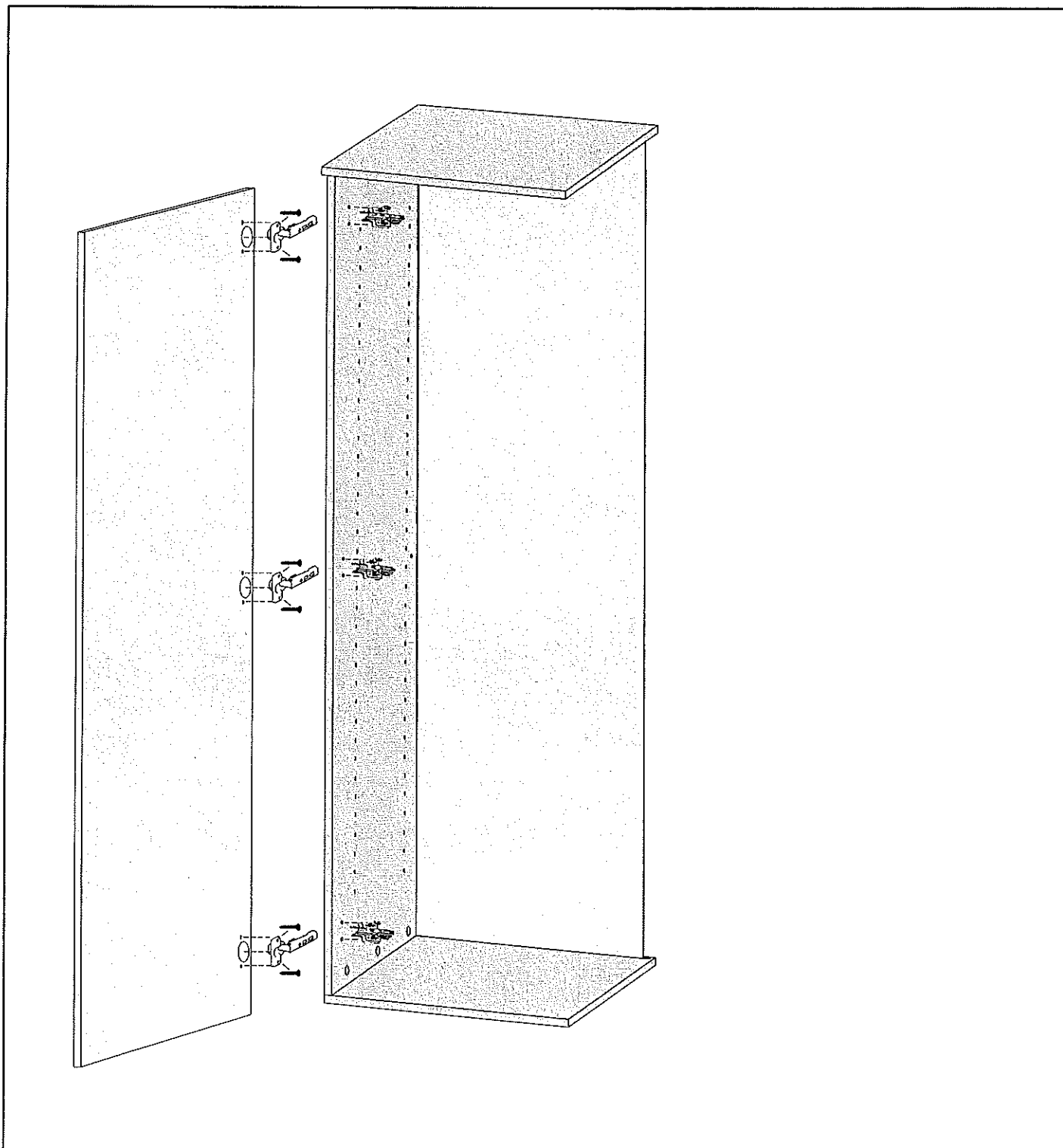
209466 ( Topfband 155° )
