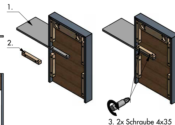
Paneel rechts mit Glasboden 155046: Ansicht von hinten (links spiegelbildlich)
