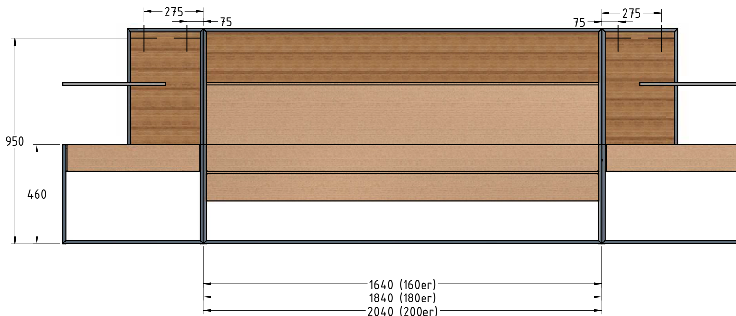
Paneel rechts mit Glasboden 155046: Ansicht von hinten (links spiegelbildlich)
