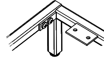
DETAY A ÖLÇEK 1 : 4
