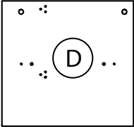
TR1976 390x407,5x16mm
