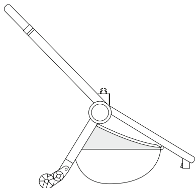
Gestell | frame
