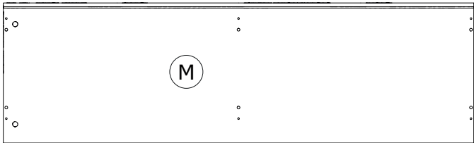
CA3841 1350x405x30mm
