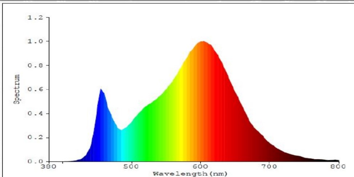
Model: 97260 (3000K)
