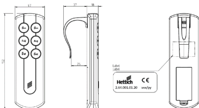
Abb. 11: Fernbedienung Funk
