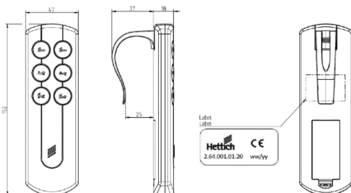
Abb. 11: Fernbedienung Funk
