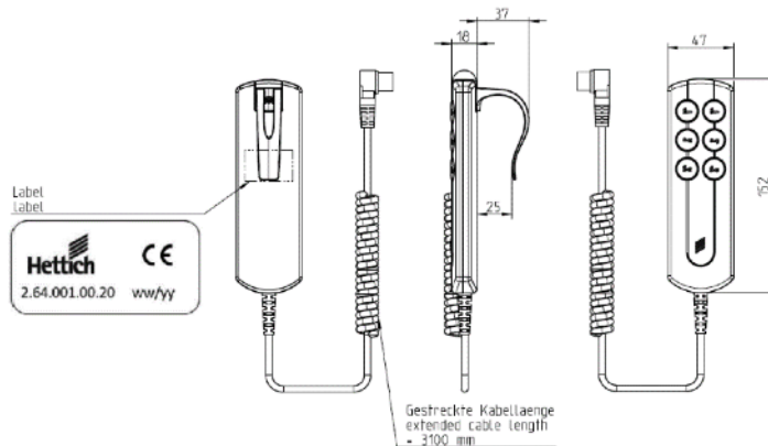
Abb. 10: Fernbedienung Kabel
