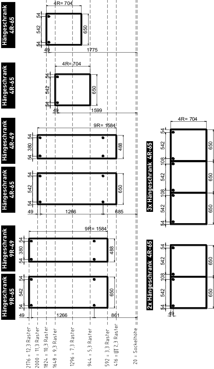
Bohrbilder Hängeschränke
