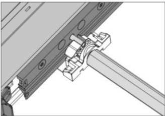
Synchronisierung Einsetzen. Placement synchroniser.
