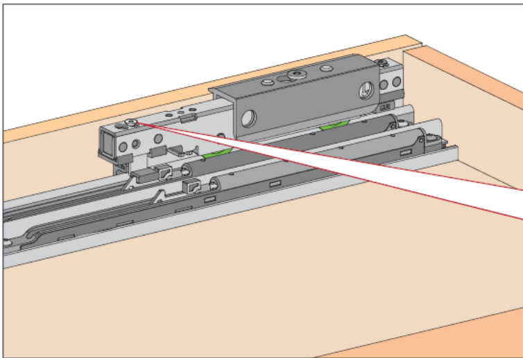
Einstellung der Sicherung. Anti-jump hook adjustment.
