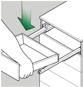
Synchronisierung Einsetzen. Placement synchroniser.
