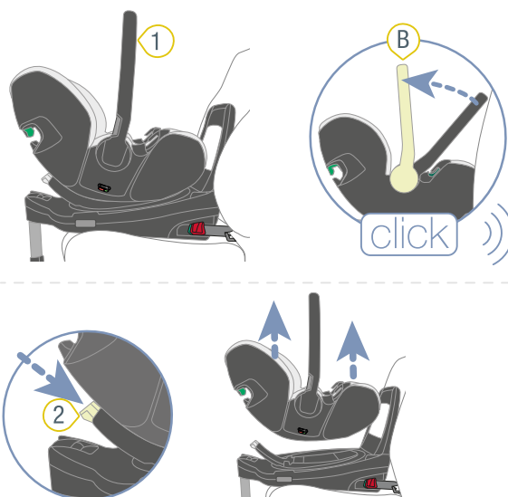
① Tragebügel
