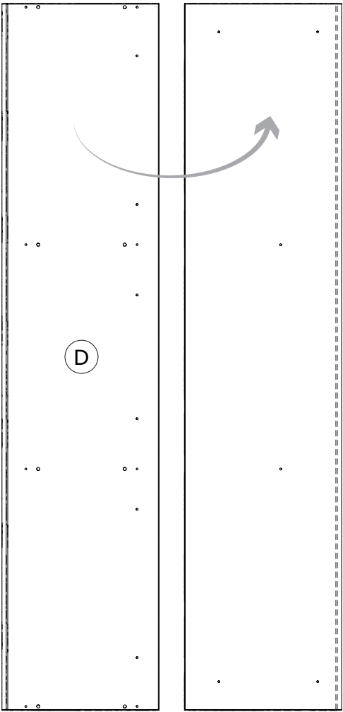
BA02511 1828x407x16mm
