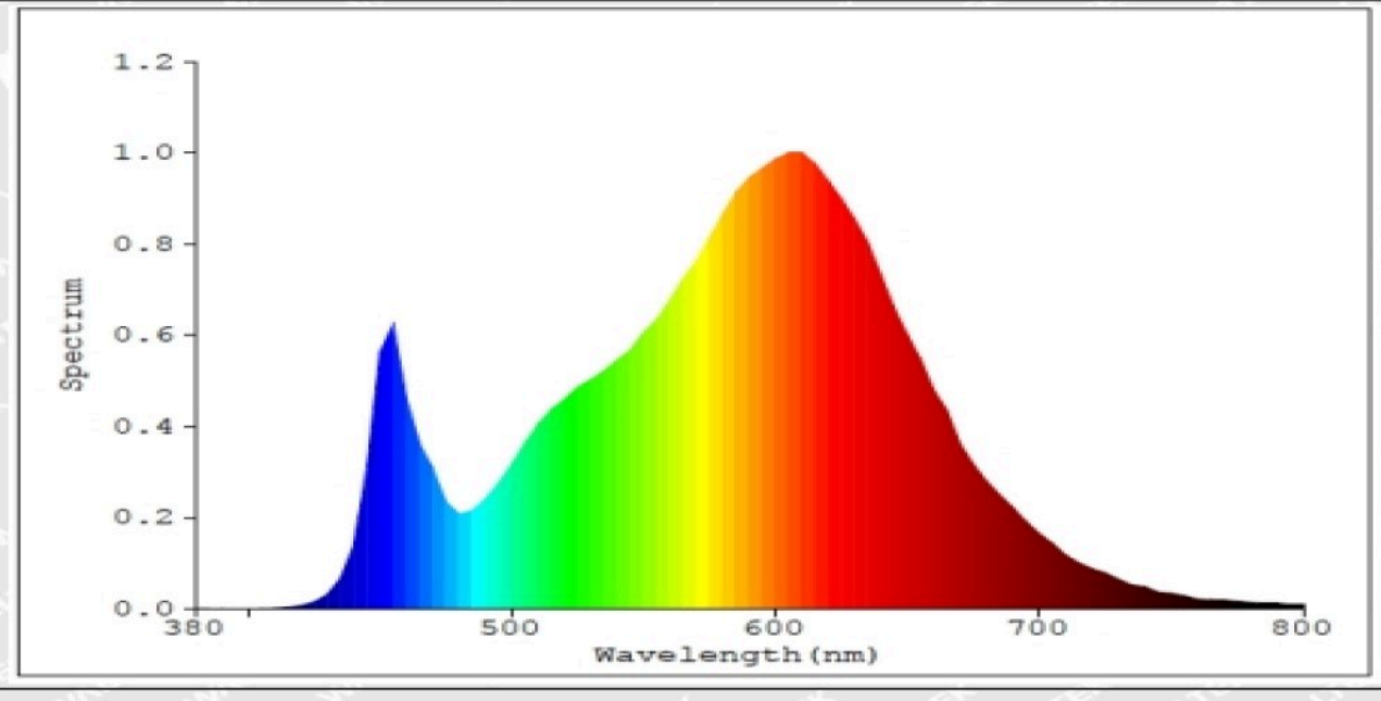
Model: 97200 (3000K)
