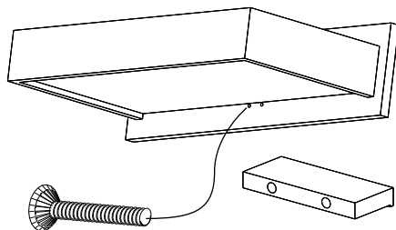
Griffe mit 2 St. „Senkschraube“ M4x25 anschrauben.
