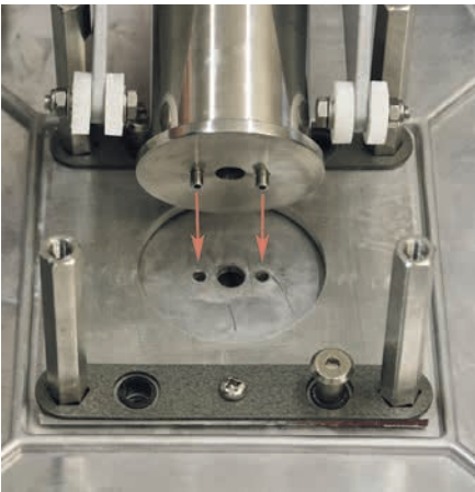
Bild/Picture 2.1 Detail ...dass die zwei Führungstifte in den Bohrungen des Ständergestells stecken
