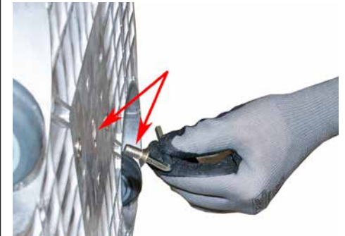
Bild/Picture 2.4 Stecken Sie die Senkschraube in die zentrale Bohrung und drehen Sie diese mit dem Sechskantschlüssel fest an. Achtung: Die Führungstifte des Aufnahmerohres müssen in den Bohrungen sein.
