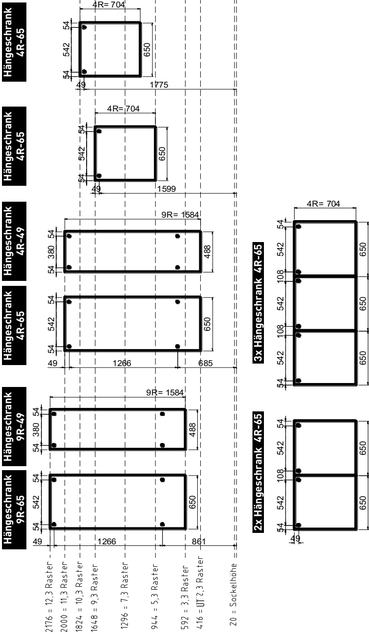
Bohrbilder Hängeschränke
